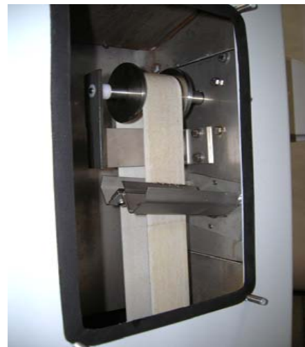
bandskimmer
